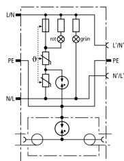
Schéma vnitřního zapojení DPRO 230 TV
