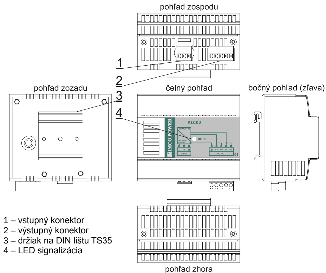
Obr.1 – mechanická konštrukcia zdroja ALC02
